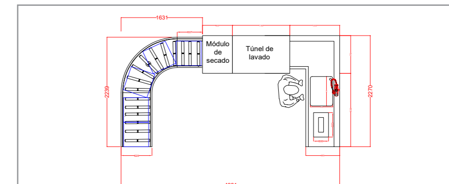
EJEMPLO DE INSTALACIÓN DESARROLLADA SEGÚN NECESIDADES DEL CLIENTE
